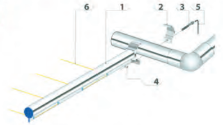
Alüminyum Küpeşte İçin Kullanıcı Montaj Şeması
